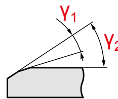
Исполнение фаски PN
